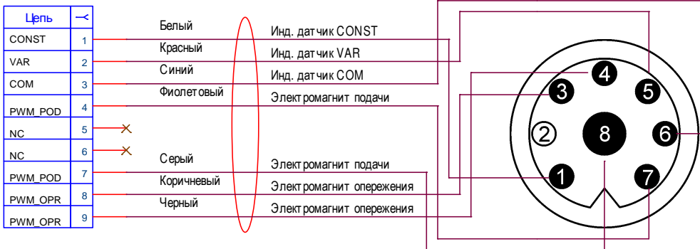
Рисунок 16. Схема распайки разъема ТНВД тип 1
