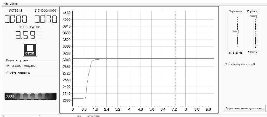
Рисунок 9. График нормально работающего насоса
