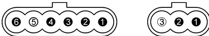
Рисунок 19. Разъем ТНВД тип 3: а – опережение и индуктивный датчик, б – катушка подачи
