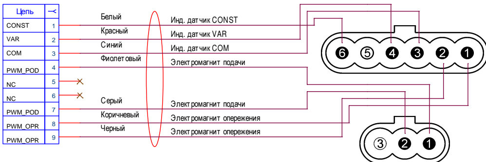
Рисунок 20. Схема распайки разъемов ТНВД тип 3
