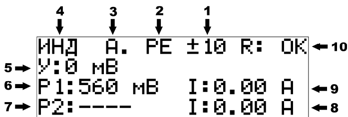
Рисунок 3. Описание информации на индикаторе прибора режим PE
