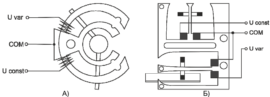
Рисунок 33. Индуктивные датчики положения рейки: а – для насоса типа VE, б – для насоса типа PE
