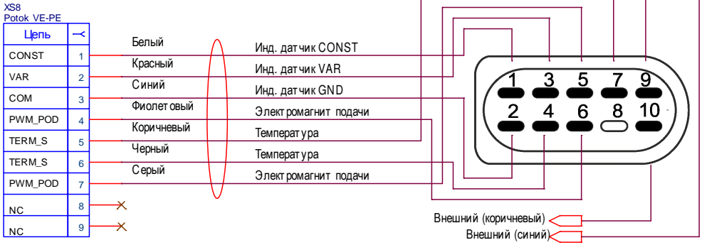
Рисунок 30. Разъем ТНВД тип 7
