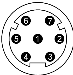
Рисунок 20. Разъем ТНВД тип 2
