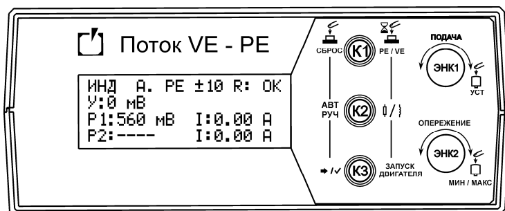
Рисунок 1. Панель передняя
