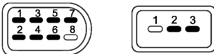
Рисунок 31. Разъем ТНВД тип 8: а – подача и индуктивный датчик, б – клапан опережения
