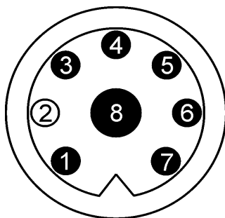
Рисунок 18. Разъем ТНВД тип 1
