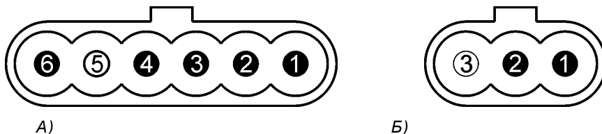
Рисунок 22. Разъем ТНВД тип 3: а – опережение и индуктивный датчик, б – катушка подачи
