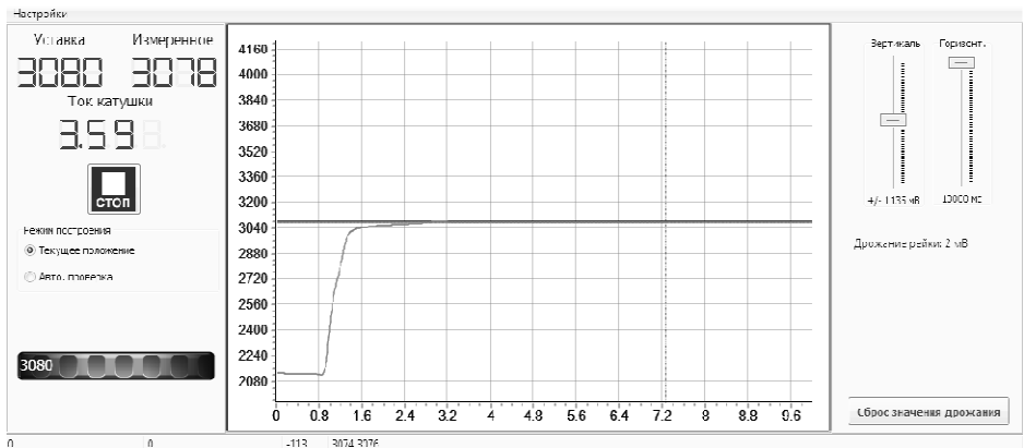
Рисунок 11. График нормально работающего насоса
