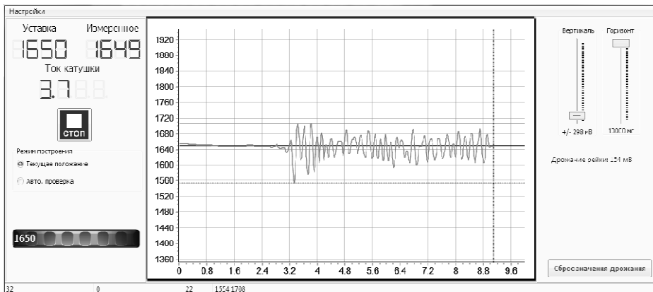
Рисунок 12. График дрожания рейки
