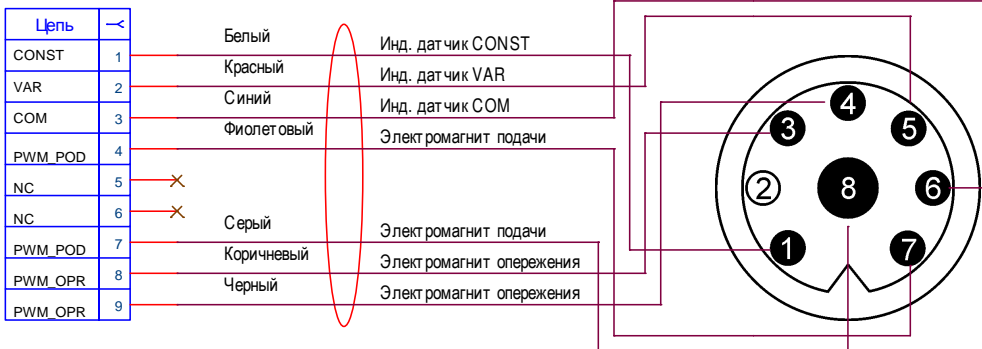
Рисунок 19. Схема распайки разъема ТНВД тип 1
