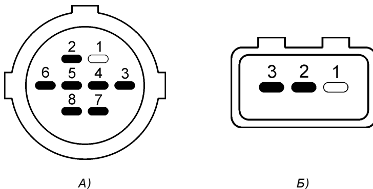
Рисунок 25. Разъем ТНВД тип 5: а – подача и индуктивный датчик, б – клапан опережения
