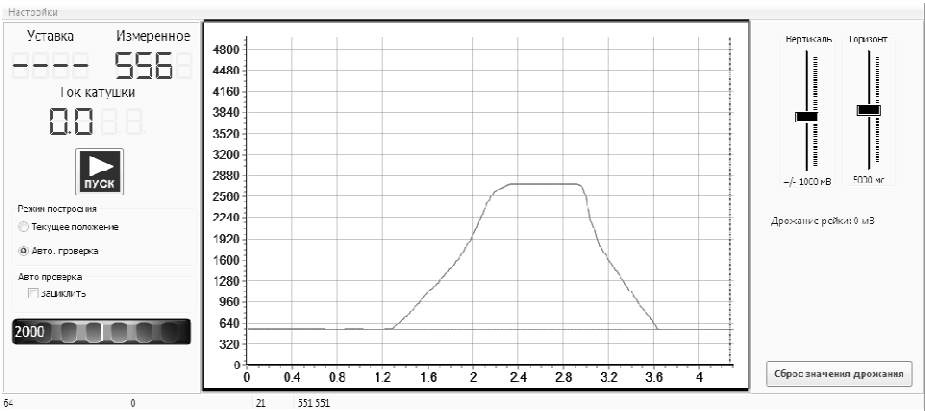
Рисунок 14. График проверки перемещения рейки насоса в автоматическом режиме на неисправной централизации VE
