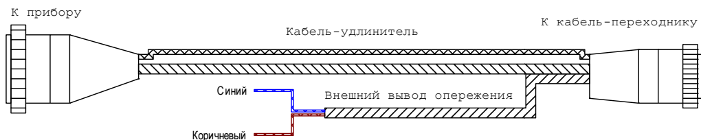
Рисунок 36. Кабель-удлинитель
