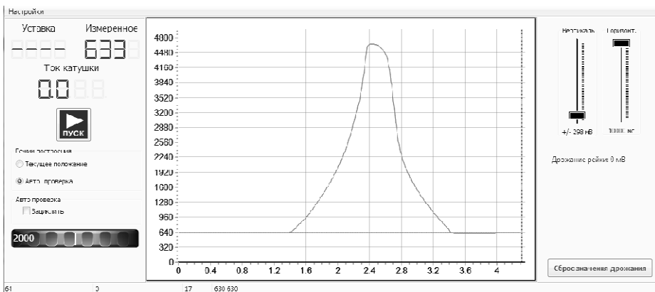
Рисунок 13. График проверки перемещения рейки насоса в автоматическом режиме на исправной централизации VE
