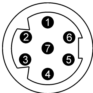
Рисунок 27. Разъем ТНВД тип 6: а – подача и индуктивный датчик, б – клапан опережения
