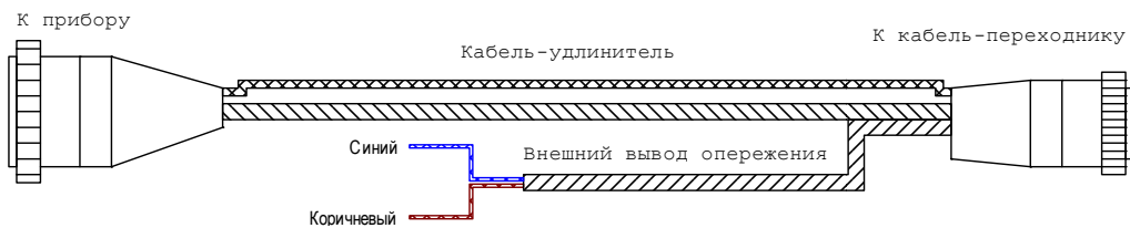
Рисунок 18. Кабель-удлинитель
