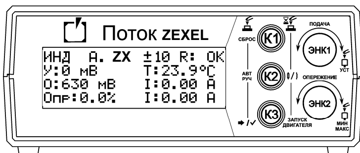
Рисунок 1. Панель передняя
