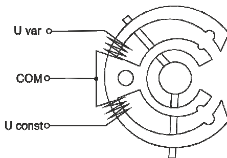
Рисунок 17. Индуктивные датчики положения рейки
