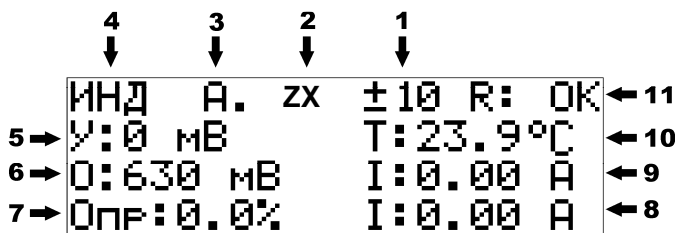
Рисунок 3. Описание информации на индикаторе прибора режим ZEXEL
